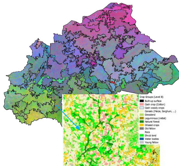
Figure 1. Agro-paysages du Burkina Faso obtenus par segmentation de série temporelle d'images Modis (sur fond de composition colorée de Composantes Principales), et zoom sur l'utilisation agricole des sols obtenue par classification orientée objet d'une série temporelle Sentinel 2 et d'une image THRS Spot 6.
