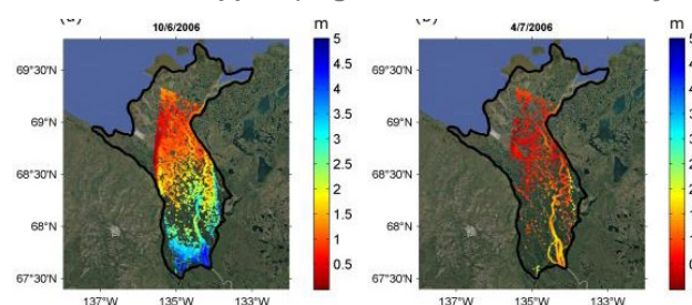
Evolution temporelle des hauteurs d'eau de surface dans le delta du McKenzie au cours de l'été 2006 (Normandin et al., 2018).
