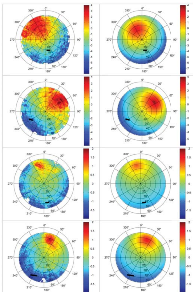
Grappe polaire montrant l'amplitude du hot spot thermique en bande large pour de l'urbain (haut) et une forêt de pins (bas) et 2 positions solaires. Le signal mesuré (gauche) est comparé au signal simulé avec le modèle RL (droite). (d'après Duffour et al., RSE, 2016)
