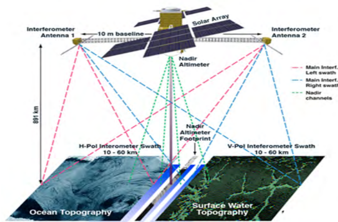
Mode de fonctionnement de Swot
