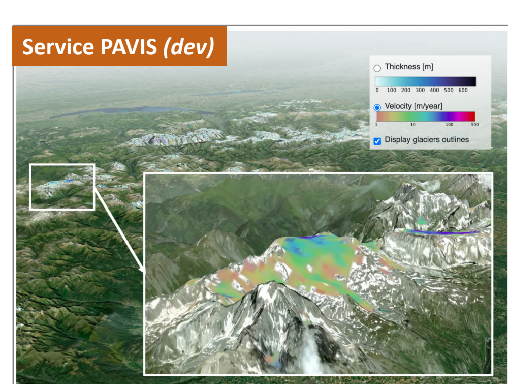
Production Automatique et Massive des Vitesse d'Écoulements des Glaciers par Imagerie Satellites
