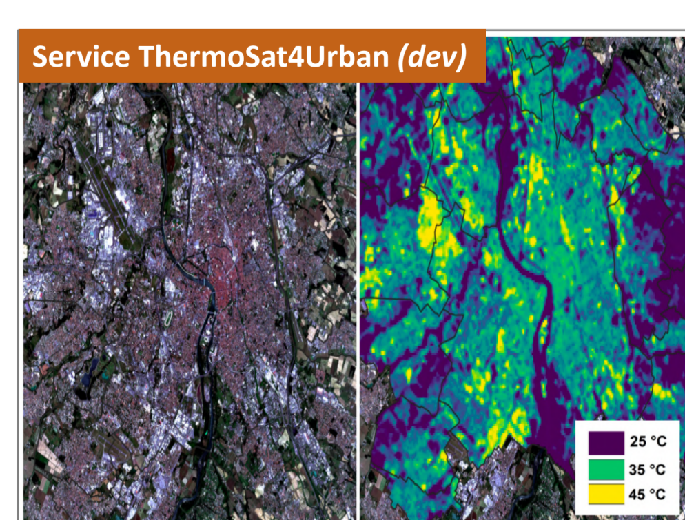
Production de températures de surface (LST) à 90 m et 30 m à partir de données ASTER.
